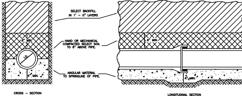
CLASS B LONGITUDINAL SECTION
