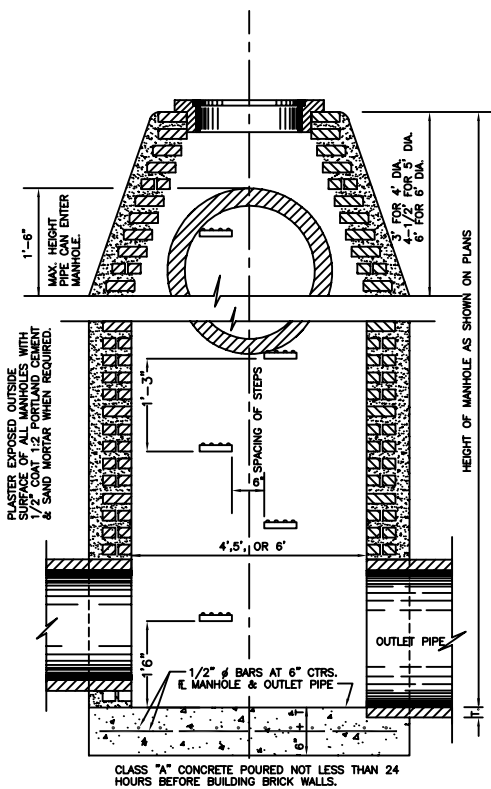
ELEVATION
